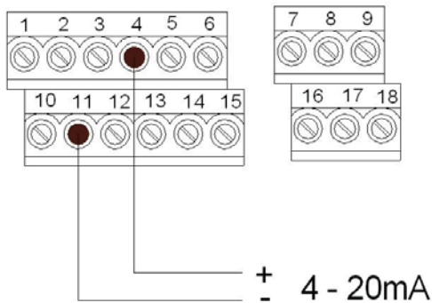
Klemmenbelegung / Terminals Controlmodule Stattox 501
