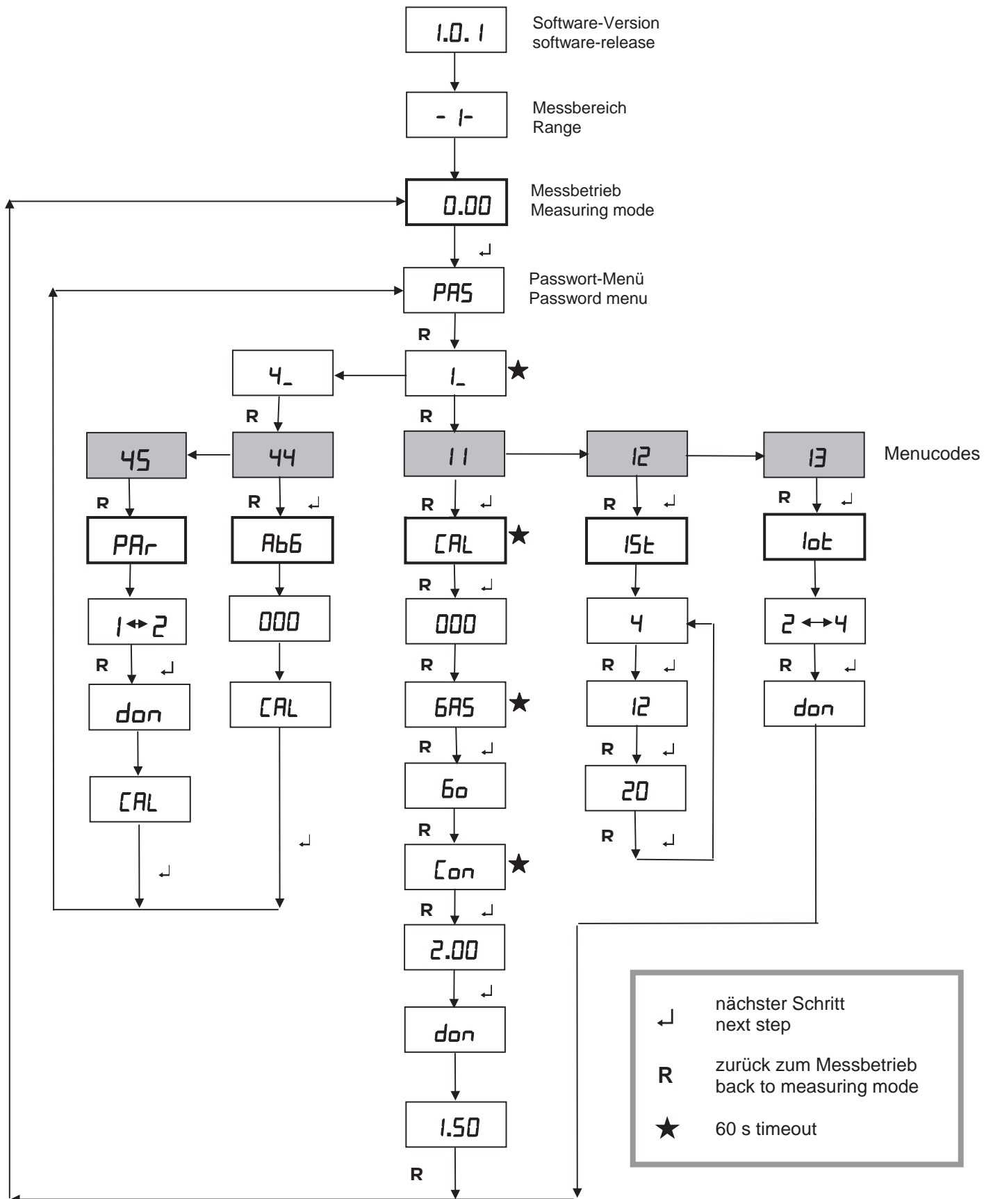
Ablaufdiagramm / Menu diagramm
